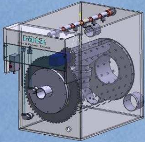
Trommelfilter
